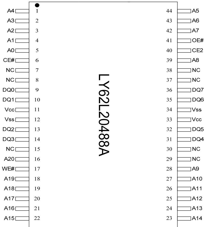
TSOP-II
