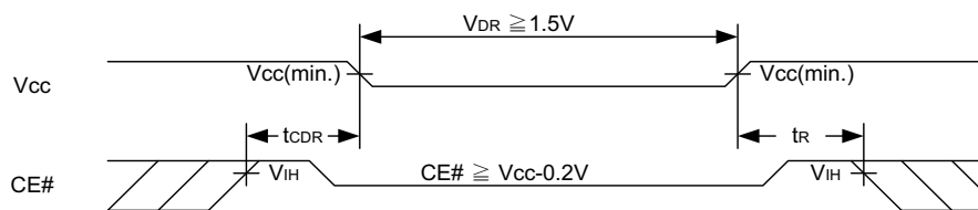
データ保持タイミング・チャート 1 (CE#コントロール)
