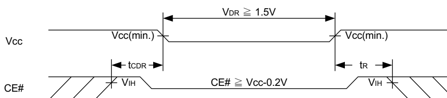
データ保持タイミング・チャート 1 (CE# コントロール) \leq
