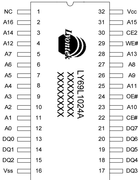
SOP
